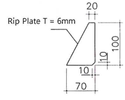
Det. Rip Plate SCALE 1 : 25
