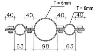
Det 4. Klem Ornamen SCALE 1 : 25
