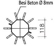
Det 2. Klem Anti Panjang SCALE 1 : 25
