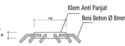
Det 2. Klem Anti Panjang SCALE 1 : 25
