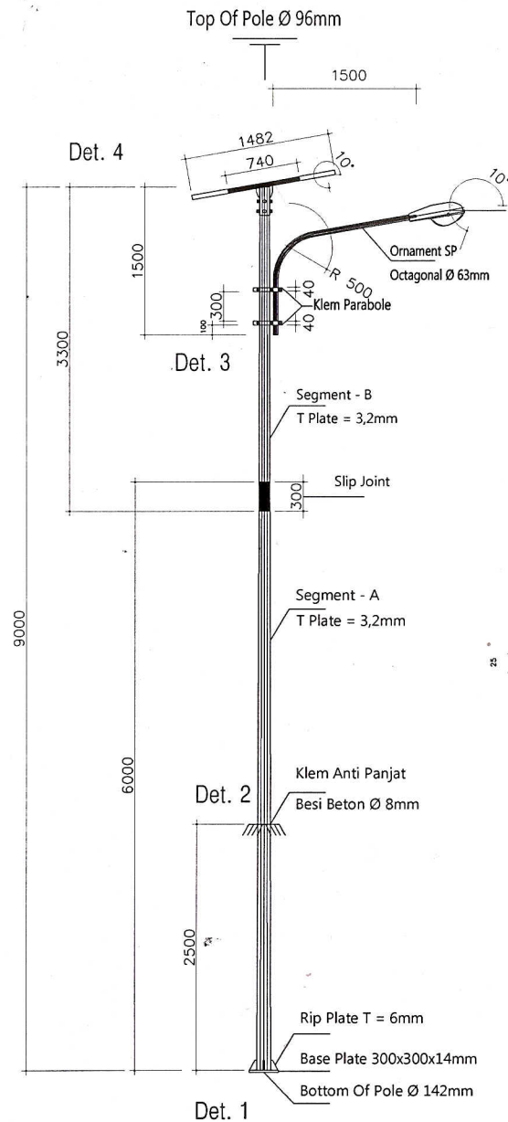
SCALE 1 : 100
