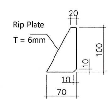
Det. Rip Plate SCALE 1 : 25
