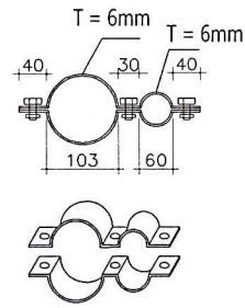
Det 4. Klem Ornament Lampu SCALE 1 : 25
