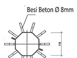
Det 2. Klem Anti Panjang SCALE 1 : 25
